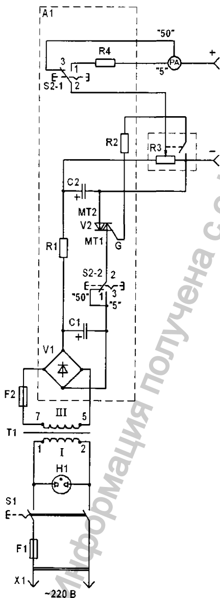
Рисунок 2 – Схема электрическая принципиальная
